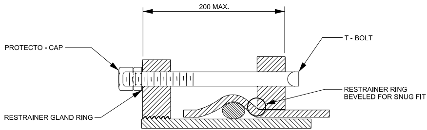
DETAIL RESTRAINER ASSEMBLY N.T.S.
